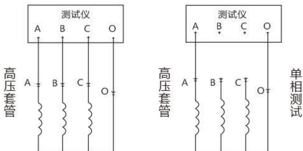
变压器绕组连接方式 - YO型
