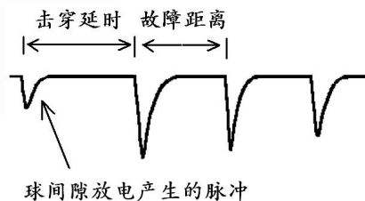
图 4-2-4 冲闪法波形
