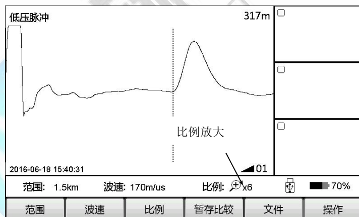
图 3-3-3 波形放大
