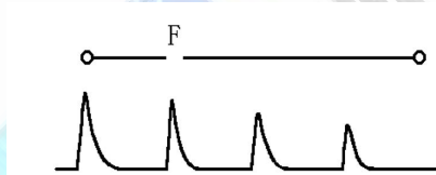
图 3-2-2 断线故障反射波形
