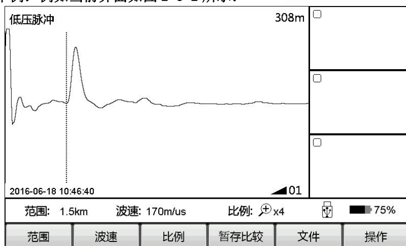
图 2-3-2 操作界面
