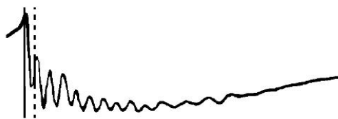
(c) 近距离故障直闪法波形
