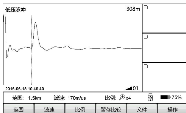
图 3-3-2 低压脉冲典型波形
