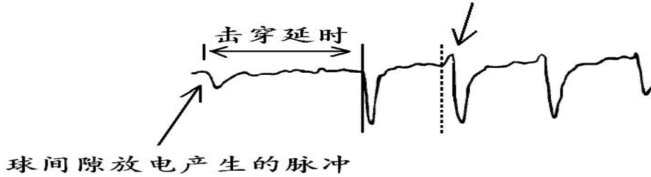
(a) 典型的冲闪法波形
