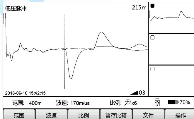
图 3-3-5 波形比较
