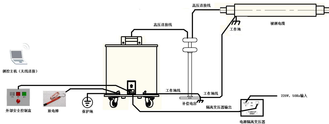
图6-6 HZZDB-30系统连接示意图（有补偿电容）
