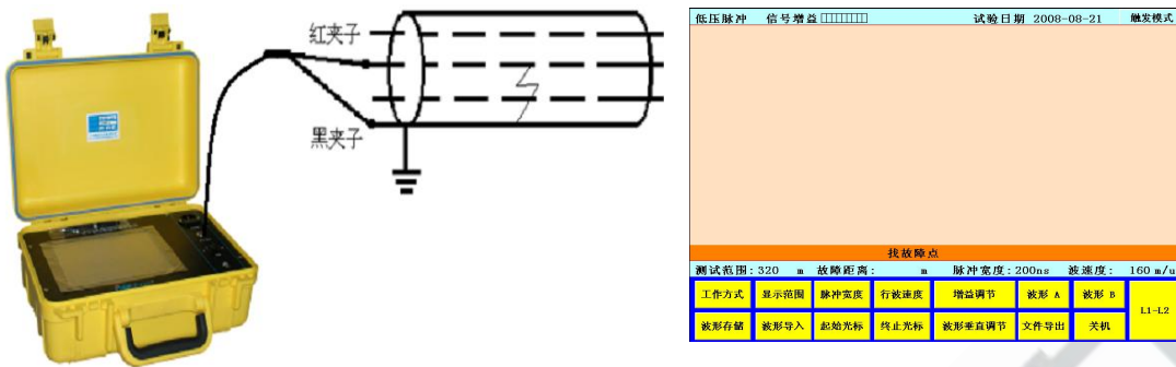
图6-2 HZTDR连接和启动界面
