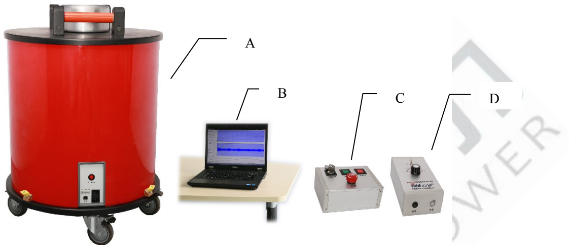
图4-1 HZZDB-30系统构成
