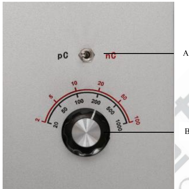
图 4-4 HZCAL-100 标准放电脉冲校准器面板 A、量程选择开关 B、档位选择旋钮
