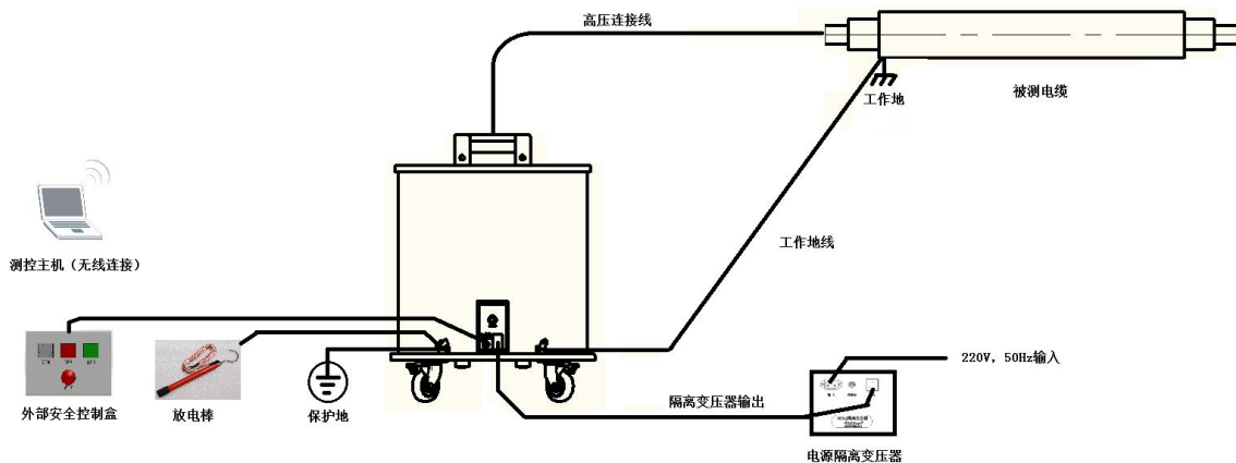
图6-5 HZZDB-30系统连接示意图（无补偿电容）
