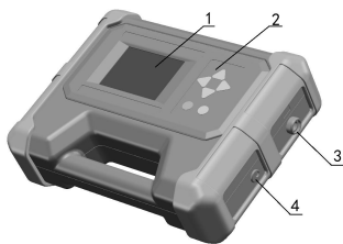
图 1-4-1 发射机整体
