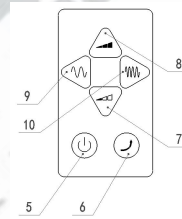
图 1-4-2 发射机键盘
