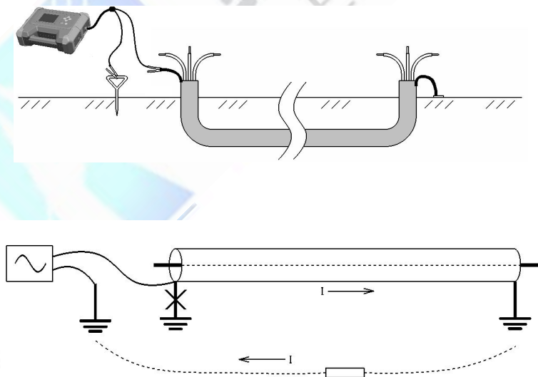
图 3-1-2 护层—大地接线法
