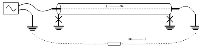
图 3-1-1 芯线—大地接线法
