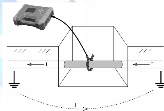
图 2-2-2 卡钳耦合法
