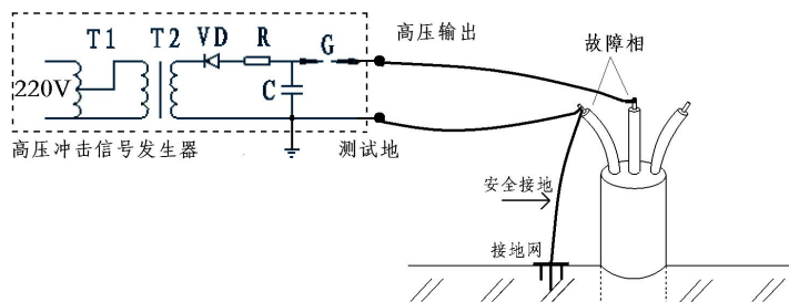
图 4-2-2 相间接法
