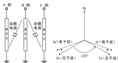
图 2 相间干扰
