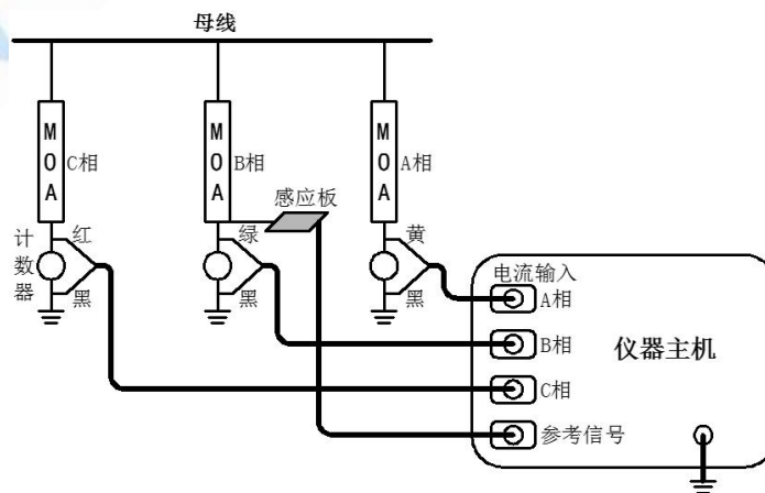
图 20 感应测试方式接线示意图（三相同步测量）
