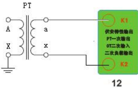
4. 接线图：图四 （PT 伏安接线图）
