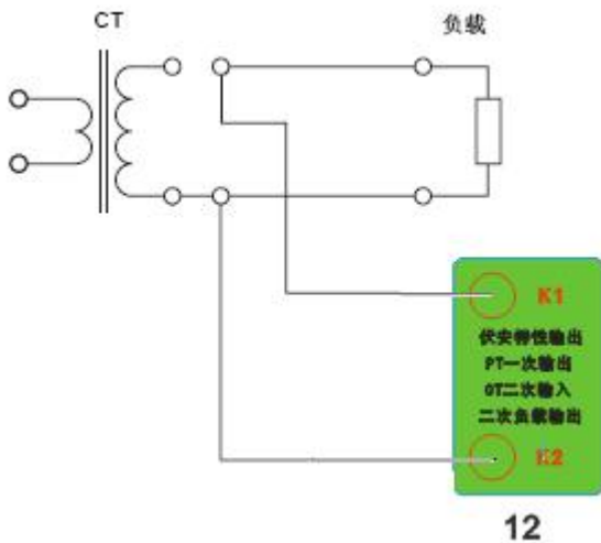
8. 接线图：图八 （二次负载接线图）
